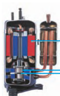
Компрессор (двухроторный)
